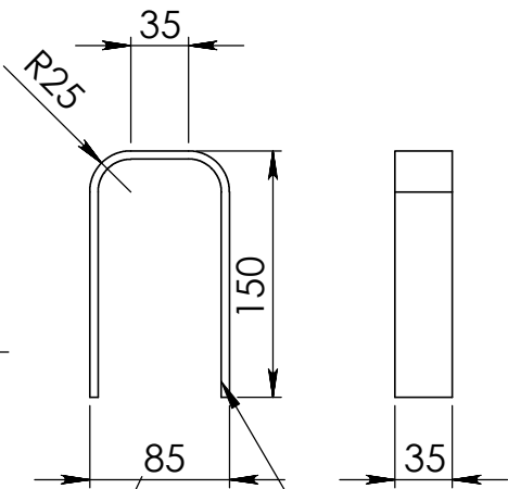
lame de ressort 35x5mm s'insère à l'intérieur(3) Echelle: 1:5
