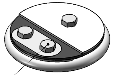
M8 boulon soudés
