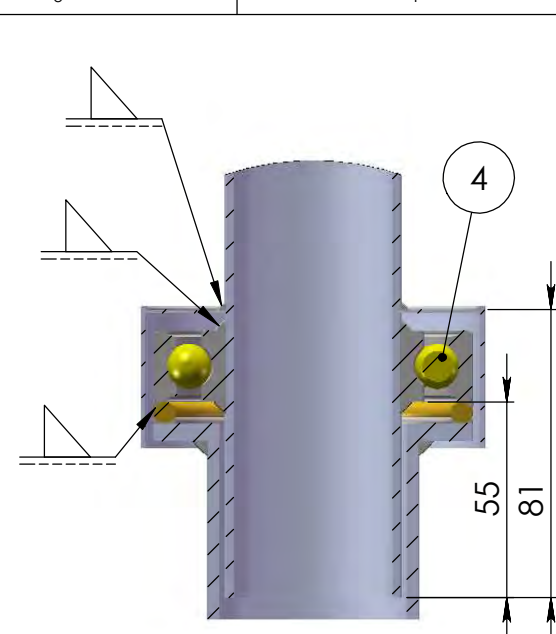
DETAIL C ECHELLE 1 : 2
