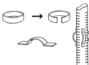
Centreurs artisanaux attachés à la crépine
