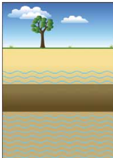
Différents aquifères
